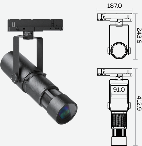
GOBO Version (Unit:mm)
